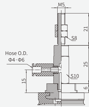
Suction cup 4×30 5×30 6×30 8×30
