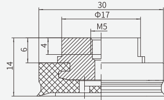
Suction cup 4×30 5×30 6×30 8×30
