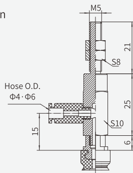
Suction cup 3.5×7 4×10 5×10 6×10
