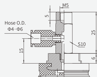
Suction cup 4×30 5×30 6×30 8×30
