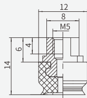
Suction cup 3.5×7 4×10 5×10 6×10
